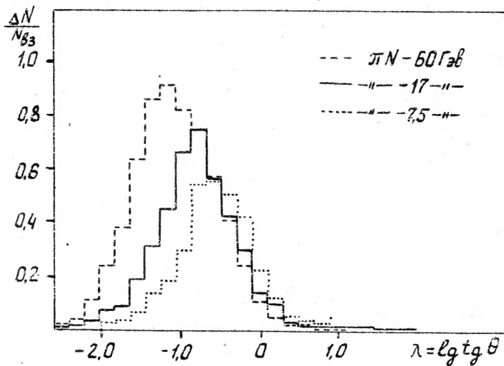
Рис. 9 б. Распределение ливневых частиц в координатах \lambda = \lg \tg \theta в \pi N взаимодействиях.
