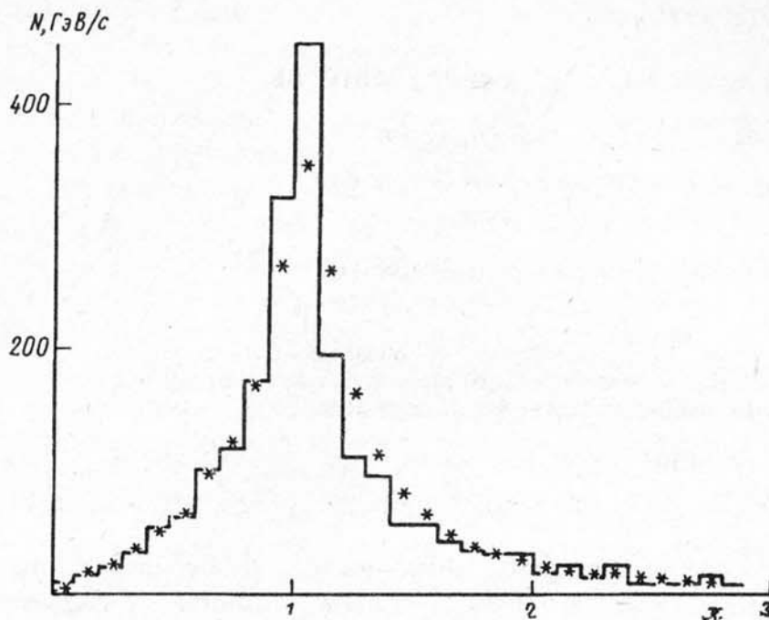
Рис.1. Распределение величины X = P_{\perp \text{эксп}}/P_{\perp \text{смм}} для протонов. Гистограмма – эксперимент, звездочки – модель независимого испускания
