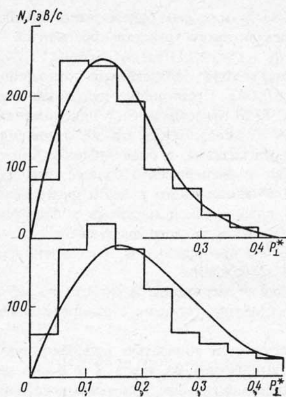
Рис.2. Распределение поперечных импульсов в СЦИ двух фрагментов. Эксперимент – нижняя гистограмма, Монте-Карло – верхняя гистограмма. Плавная кривая – ожидаемое распределение Рэлея
