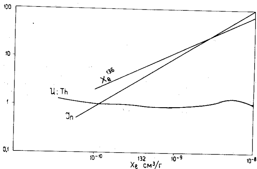
Рис. 4. Относительное изменение U, Th, Jh и ^{136}\text{Xe} с ростом ^{132}\text{Xe} .
