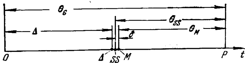
Рис. 3. Временная шкала нуклеосинтеза и образования Солнечной системы. 0 - начало нуклеосинтеза, Δ - конец нуклеосинтеза, т.е. последний момент, когда r-процесс дает вклад в образование материала Солнечной системы, SS - образование Солнечной системы, M - образование метеоритов и Земли, P - настоящий момент.
