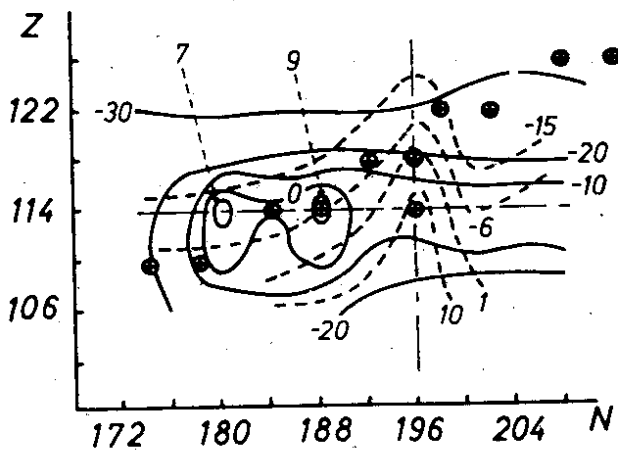
Рис. 1. Ожидаемые периоды полураспада СТЭ, \log \tau /лет/.
