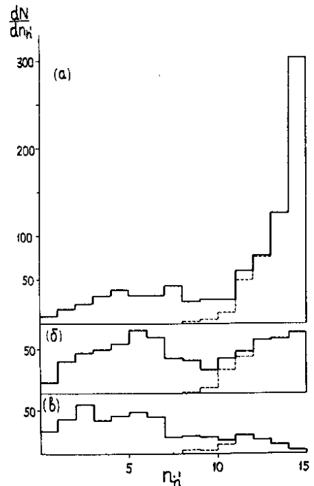
Рис. 4. Распределения по множественности h' -частиц, испущенных ^{28}\text{Si} во взаимодействиях с ядрами \text{AgBr} (а), \text{CNO} (б) и \text{H} (в). Пунктиром выделены события ПР.
