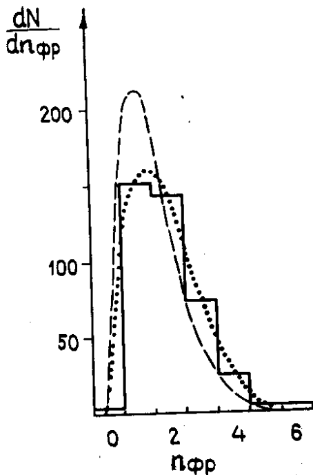
Рис. 5. Распределение по зарядам фрагментов во взаимодействиях ^{28}\text{Si} с нуклонами. Гистограмма – эксперимент, точки – расчет по модели перколяции с параметрами p=0,55 (штриховая линия) и p=0,6 (пунктир). Нормировка по площади. Кривые, соединяющие точки, проведены от руки.
