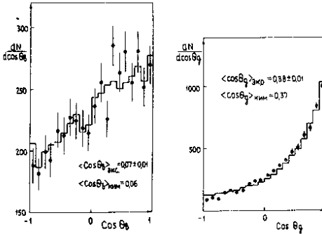
Рис. 5. Распределения по \cos \theta для b- и g-частиц. Обозначения те же, что на рис. 4.
