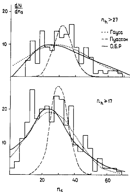
◀ Рис. 2 Распределения по множественностям s-частиц для событий с n_h \geq 17 и n_h > 27 .
