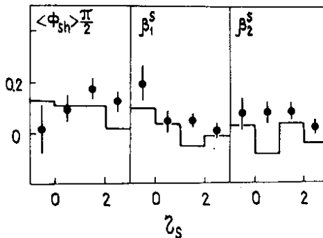
Рис. 11. Зависимость \langle \Phi_{sh} \rangle , \langle \beta_1^s \rangle и \langle \beta_2^s \rangle от псевдобыстроты \eta_s .
