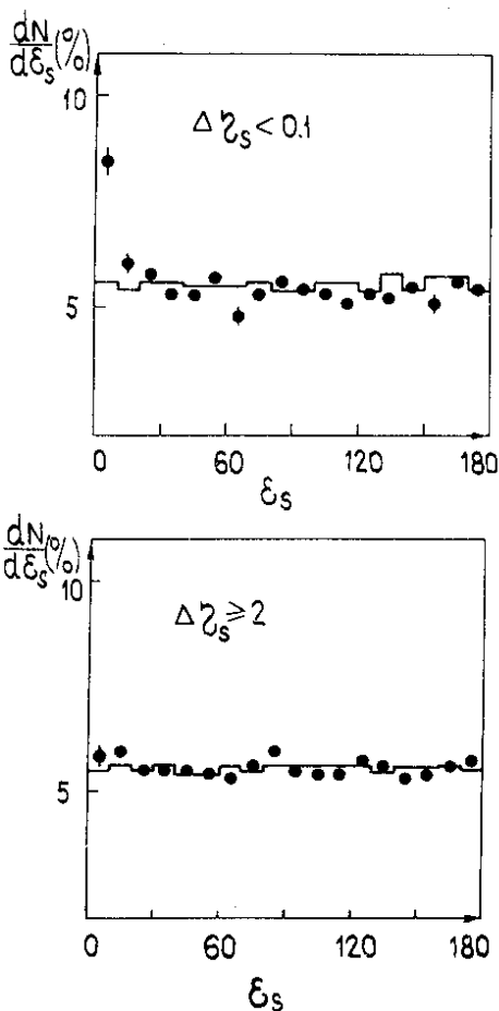
Рис. 10. Распределение по парному азимутальному углу \epsilon . Точки - эксперимент, гистограмма - КИМ.
