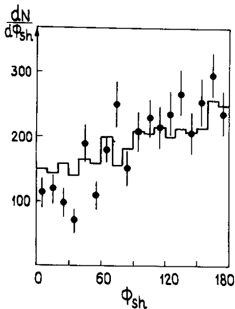
Рис. 9. Распределение по углу между результирующими векторами s - и n -частиц в азимутальной плоскости.
