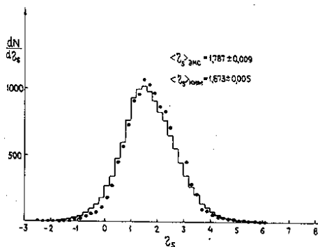
Рис. 4. Распределения по псевдобыстроте \eta_s = -\ln \operatorname{tg} (\theta/2) для всех взаимодействий. Точки – эксперимент, гистограмма – КИМ.
