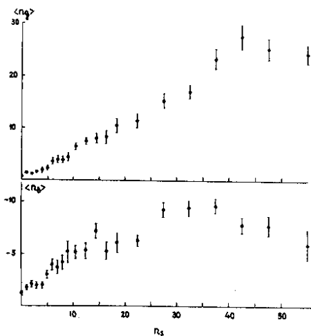
◀ Рис. 2 Распределения по множественностям s-частиц для событий с n_h \geq 17 и n_h > 27 .
