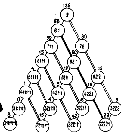
Рис.4. Схема двухтелных распадов с испусканием одно- или двухзарядной частицы из спектаторной части ядра-снаряда.
