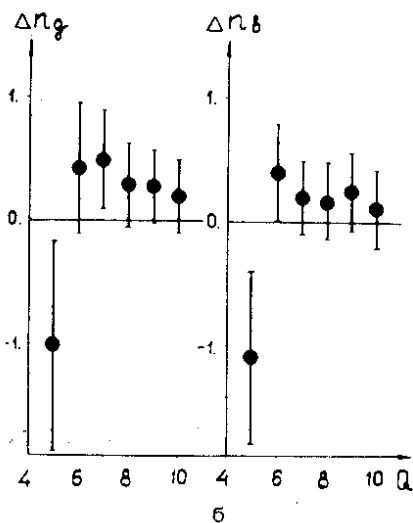
Рис.5. Средние множественности s -частиц для событий с Z_f \geq 3 и ПР в зависимости от Q/a . Разности множественностей \Delta n_g и \Delta n_b в событиях с Z_f \geq 3 и ПР /6/.
