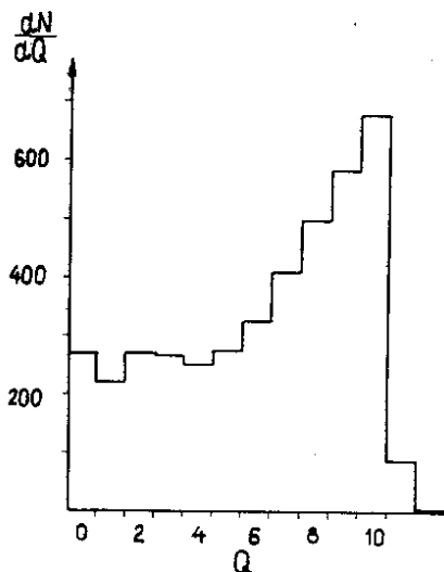
Рис.1. Распределение числа событий по суммарному заряду релятивистских фрагментов Q = \sum_i Z_f^i .
