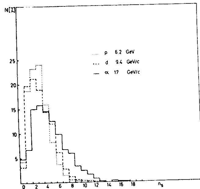
Рис. 3. Распределения по n_s для "αА-событий". Здесь же приведены данные для d-ядро/6/ и p-ядро/5/.
