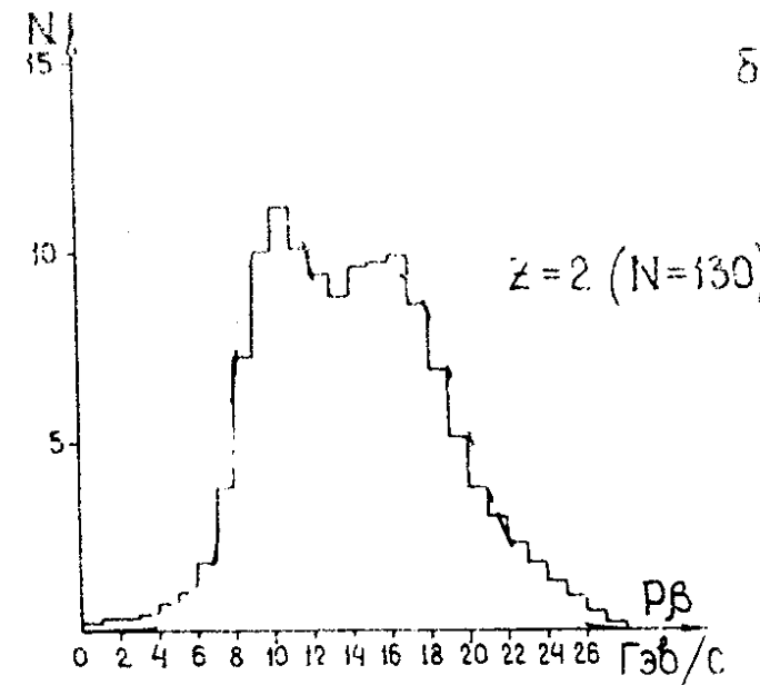
Рис. 9. а/ Распределение по p\beta для " \alpha A-1 событий" / Z=1, 0 < 3^\circ /. б/ Распределение по p\beta для " \alpha A-2 событий" / Z=2, 0 < 3^\circ /. Данные обработаны по методу работы [11].
