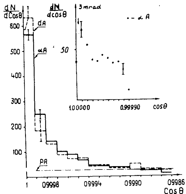
Рис. 6. Угловое распределение для "событий \alpha A-1 " / Z=1, \theta < 3^\circ /. Там же приведены распределения для d-ядро/6/ и p-ядро/8/.
