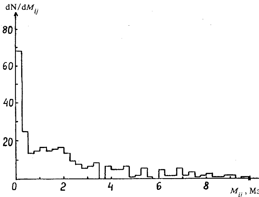
Рис.2. Распределение по разности эффективной массы пары \alpha -частиц и удвоенной массе \alpha -частиц в реакции (1)
