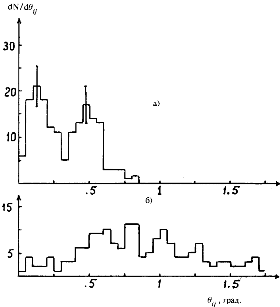
Рис.3. Распределение dN/d\theta_{ij} в л.с. для подгрупп событий с \langle p_T \rangle < 100 \text{ МэВ} (а) и \langle p_T \rangle > 100 \text{ МэВ/с} (б) (значения \langle p_T \rangle — для с.ц.м. ядра ^{12}\text{C} [1])
