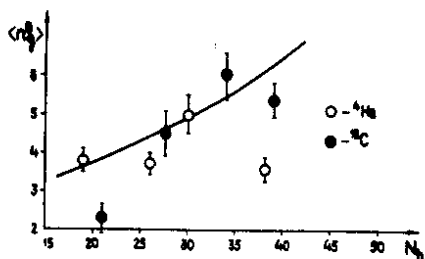
Рис.4. \langle n_g^B \rangle в зависимости от N_B для центральных столкновений. Кривая - расчет по КИМ.
