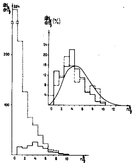
Рис.2. Распределения по числу серых адронов, вылетающих в заднюю полусферу в лабораторной системе координат - n_g^B : ... - все ^4\text{He-Ag, Br} взаимодействия, — центральные ^4\text{He-Ag, Br} взаимодействия, - - - центральные ^{12}\text{C-Ag, Br} соударения. Кривая - расчет по КИМ для центральных ^4\text{He-Ag, Br} взаимодействий.
