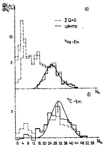
Рис. 1. Распределения по множественности сильноионизирующих h частиц. --- Q=0 ; — центральные столкновения. а/ для взаимодействий ядер {}^4\text{He} с ядрами эмульсии; ... — после вычитания событий с нейтронами-фрагментами ядра-снаряда; — для {}^4\text{He}-\text{Ag, Br} взаимодействий. б/ для взаимодействий ядер {}^{12}\text{C} с ядрами эмульсии.
