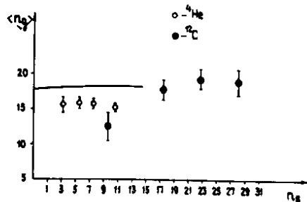
Рис.3. \langle n_g \rangle как функция n_S для центральных столкновений ядер гелия и углерода с ядрами серебра и брома. Кривая - расчет по КИМ.
