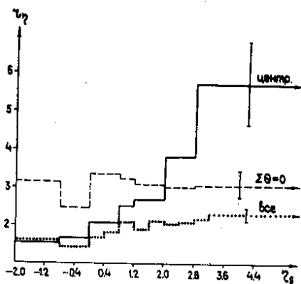
Рис.6. Отношение инклюзивных спектров \Gamma_\eta в зависимости от квазибыстроты s частиц - \eta_s .
