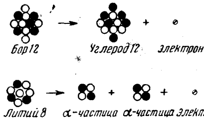
Рис. 10. Два примера изменения состава ядер при бета-распаде.
