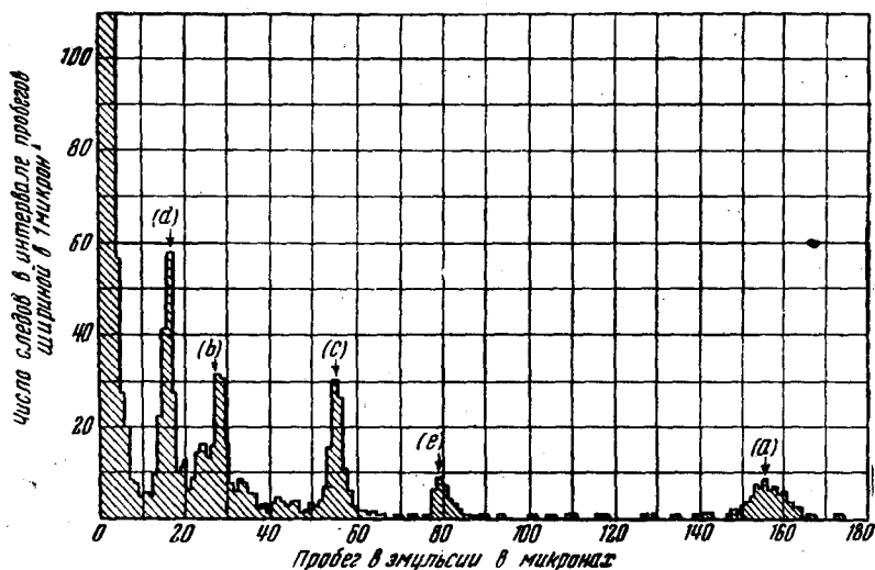
Рис. 13. Распределение по пробегам следов, получающихся при расщеплении бериллия дейтонами с энергией 900 KeV
