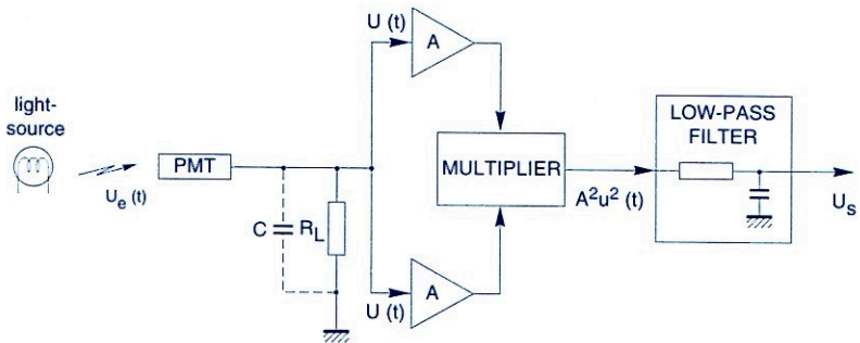
Fig.5.39 Quadratic detector
