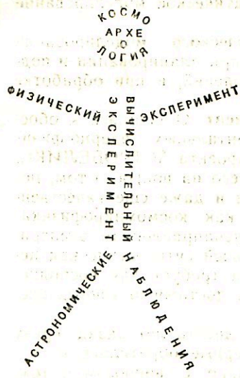
Рис. 15. Структура проекта АСТРОБЕЛИКС
