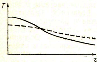
Рис. 6. При наличии космонов распределение температуры в центральной части Солнца сглаживается (штриховая линия) и температура в центре Солнца оказывается ниже, чем в стандартной модели Солнца
