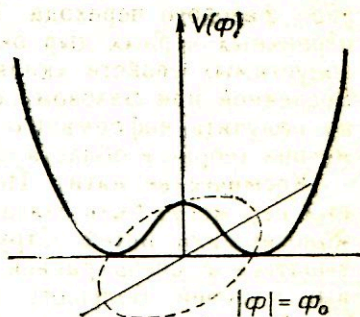
Рис. 11. Минимум потенциала V(\Phi) комплексного поля \Phi достигается в любой точке окружности |\Phi| = \Phi_0
