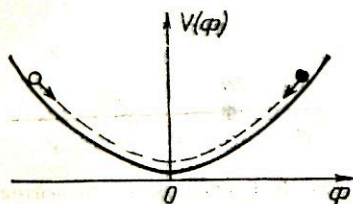
Рис. 7. При малых временах t < \hbar/mc^2 скалярное поле имеет уравнение состояния \rho = -\epsilon , а затем его колебания в окрестности минимума приводят к усредненному по периоду колебаний уравнению состояния \rho = 0
