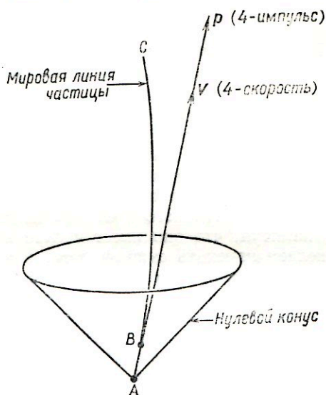
Ф и г. 15.1. 4-скорость и 4-импульс частицы.
