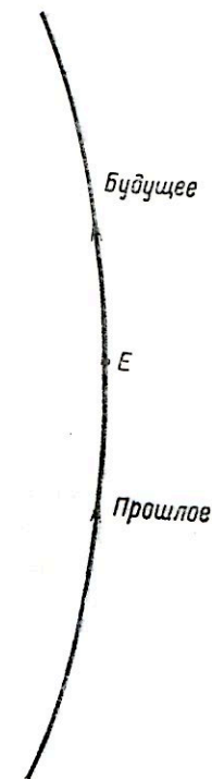
Ф и г. 7.3. Стрела времени на мировой линии частицы.
