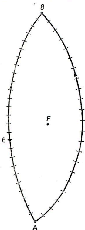
Ф и г. 9.1. Рисунок иллюстрирует понятие времени и разбирает «парадокс часов».
