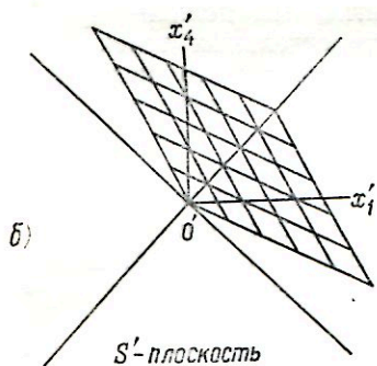
Ф и г. 14.1. Квадратная S -сетка отображается в ромбическую S' -сетку.
