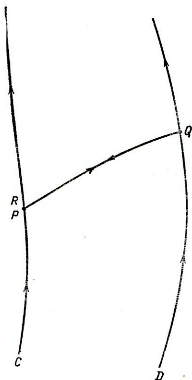
Ф и г. 7.6. Ньютоновский мгновенный сигнал.
