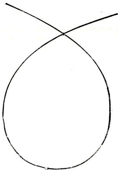
Ф и г. 7.2. Бессмыслица или нет?
