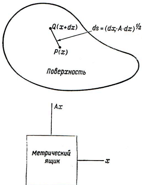
Ф и г. 10.1. Элемент длины и метрический функциональный ящик.
