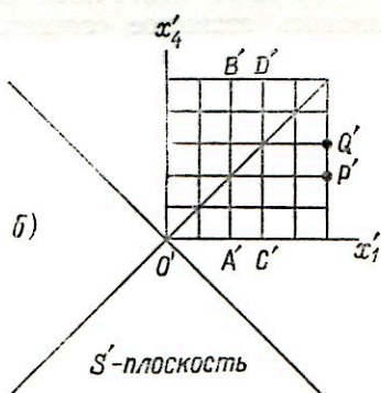
Ф и г. 14.2. Квадратная S' -сетка отображается в ромбическую S -сетку.
