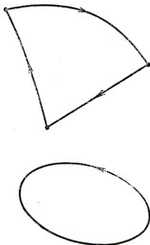
Ф и г. 7.5. Невозможные графики.
