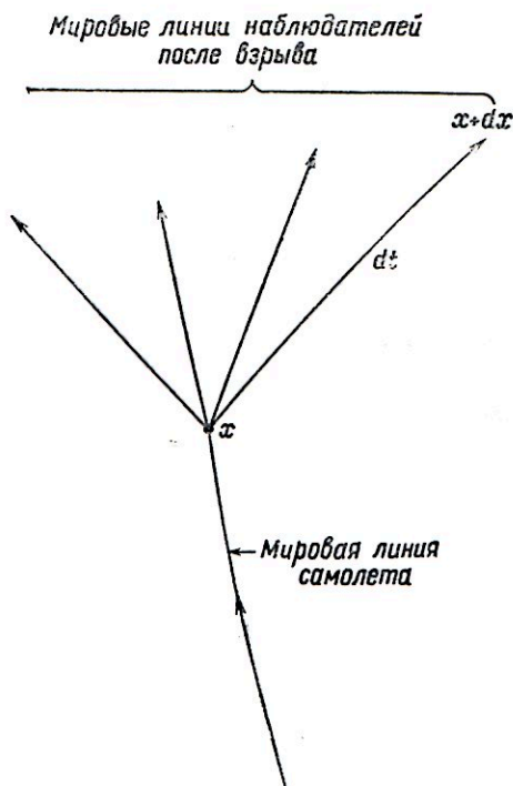
Ф и г. 11.1. Как экспериментально определить элемент длины пространства-времени.
