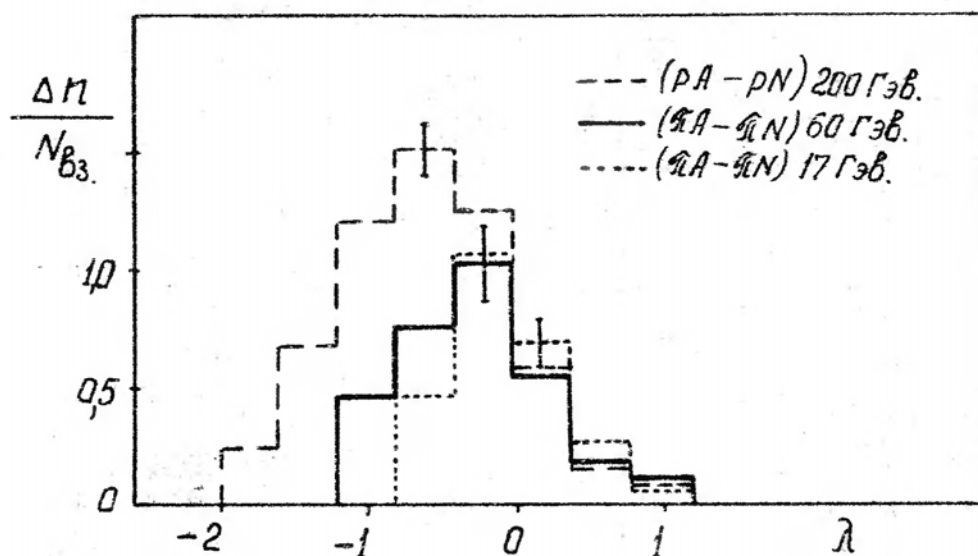
Рис. 9 а. Угловые распределения, найденные как разность распределений ливневых частиц по \lambda в адрон-ядерных и адрон-нуклонных взаимодействиях.
