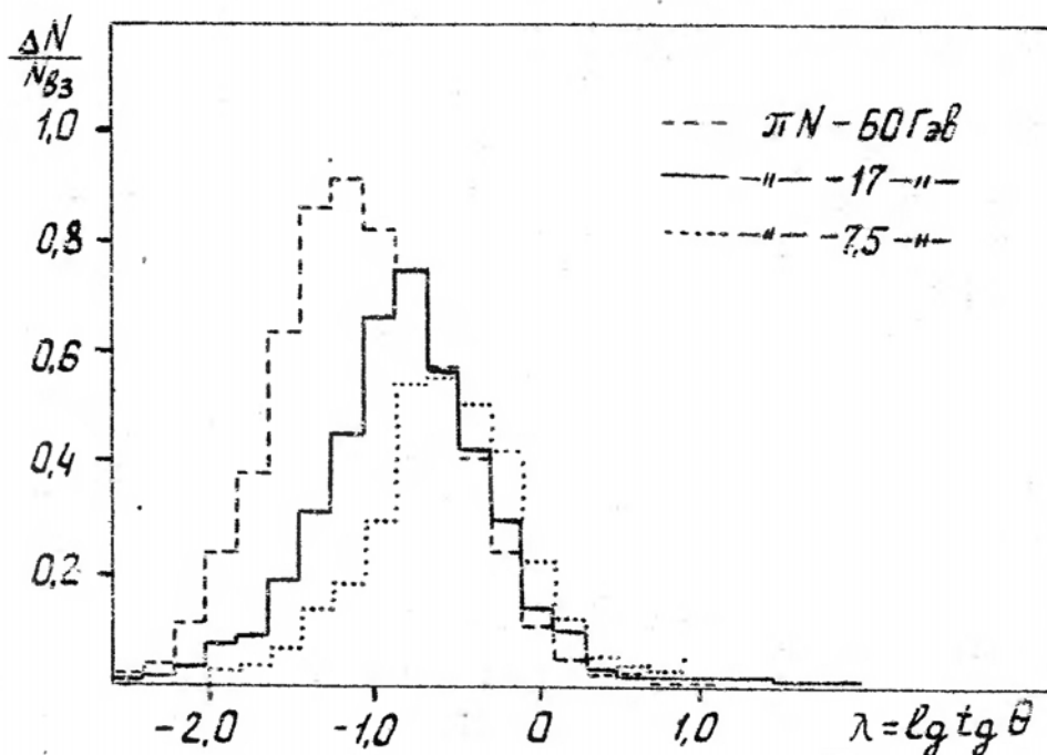
Рис. 9 б. Распределение ливневых частиц в координатах \lambda = \lg \tg \theta в \pi N взаимодействиях.
