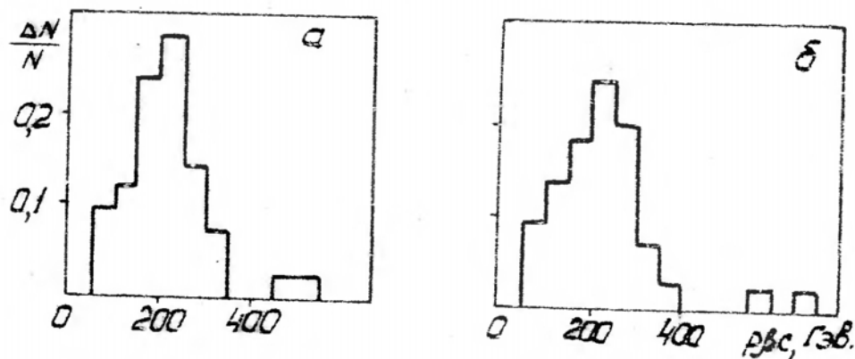
Рис. 11. Распределение по p_{\beta c} , найденных методом относительного рассеяния, на ячейках а - t = 6 мм; б - t = 8 мм.
