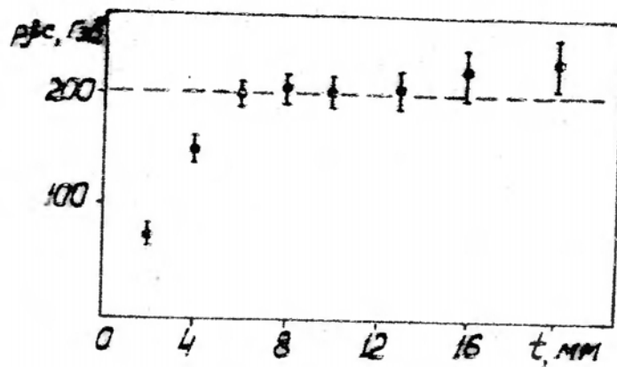
Рис. 10. Зависимость средних значений p_{\beta c} от длины ячейки.
