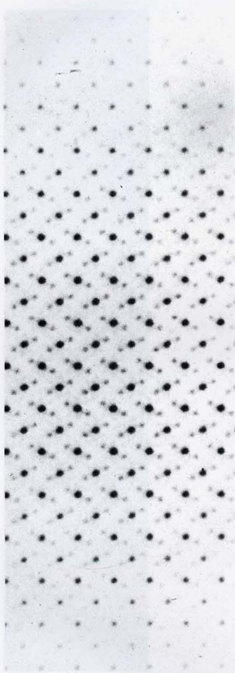
Атомы минерала марказита, увеличенные в 4,5 млн. раз в микроскопе, использующем как видимый свет, так и рентгеновские лучи. В марказите периодически повторяется группа атомов FeS_2 . Атомы железа (Fe) представлены крупными пятнами, атомы серы (S) — парами маленьких с двух сторон от крупного. С разрешения проф. М. Дж. Бюргера, Массачусетский технологический институт
