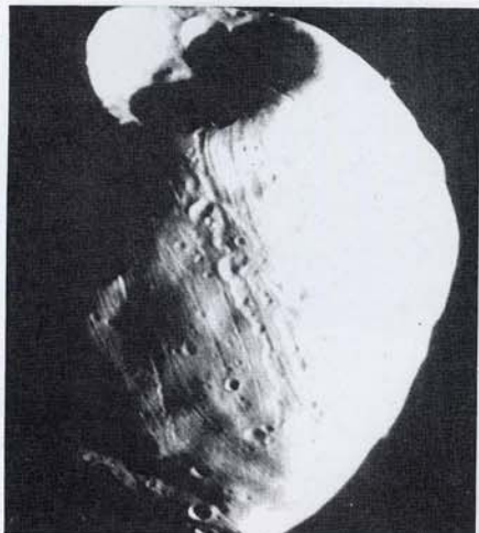
Фобос — ближайший спутник Марса. Вверху виден кратер Стикни. Если бы объект, столкновение с которым породило этот кратер, был немного крупнее, Фобос мог бы разрушиться. Снимок с орбитального аппарата «Викинг-1». С разрешения NASA
