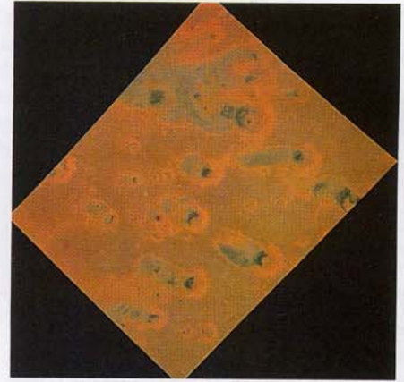
Песок и пыль, наметенные с подветренной стороны ударных кратеров на Синус Меридиани. С разрешения NASA
