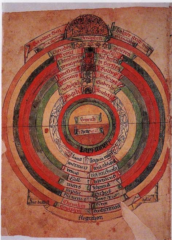
Геоцентрическая докоперниковская Вселенная христианской Европы. В центре — Земля, разделенная на Небеса (светлые) и Ад (темный). Землю окружают элементы: вода (зеленая), воздух (голубой) и огонь (красный). Далее, в направлении изнутри наружу, следуют сферы, содержащие семь планет, включая Луну и Солнце, а также «Двенадцать чинов блаженных духов», херувимов и серафимов. Из немецкого астрологического манускрипта, ок. 1450 г.
