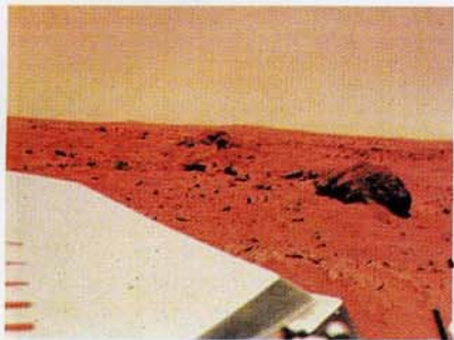
Присыпанный песком булыжник на Равнине Хриза, получивший название Большой Джо. Если бы «Викинг-1» опустился на него, то потерпел бы катастрофу. С разрешения NASA
