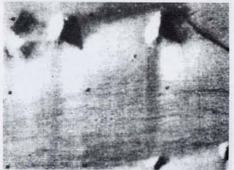
Пирамиды Элизиума. Снимок «Маринера-9». С разрешения NASA
