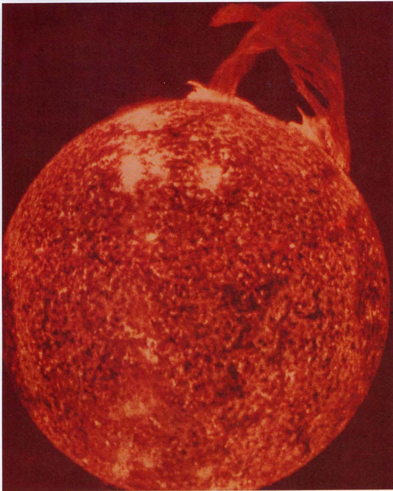
Ближайшая звезда: Солнце, видимое в далекой ультрафиолетовой линии излучения ионизированного гелия. Протуберанец вверху справа на короткое время вытянулся на 300 000 км в космос, но вскоре вновь упадет в ярко светящийся газ солнечной поверхности. Наименьшие пятна горячего газа, видимые на этом изображении солнечной поверхности, сравнимы по размерам с Землей. Фото с орбитальной станции «Скайлэб-4». С разрешения NASA
