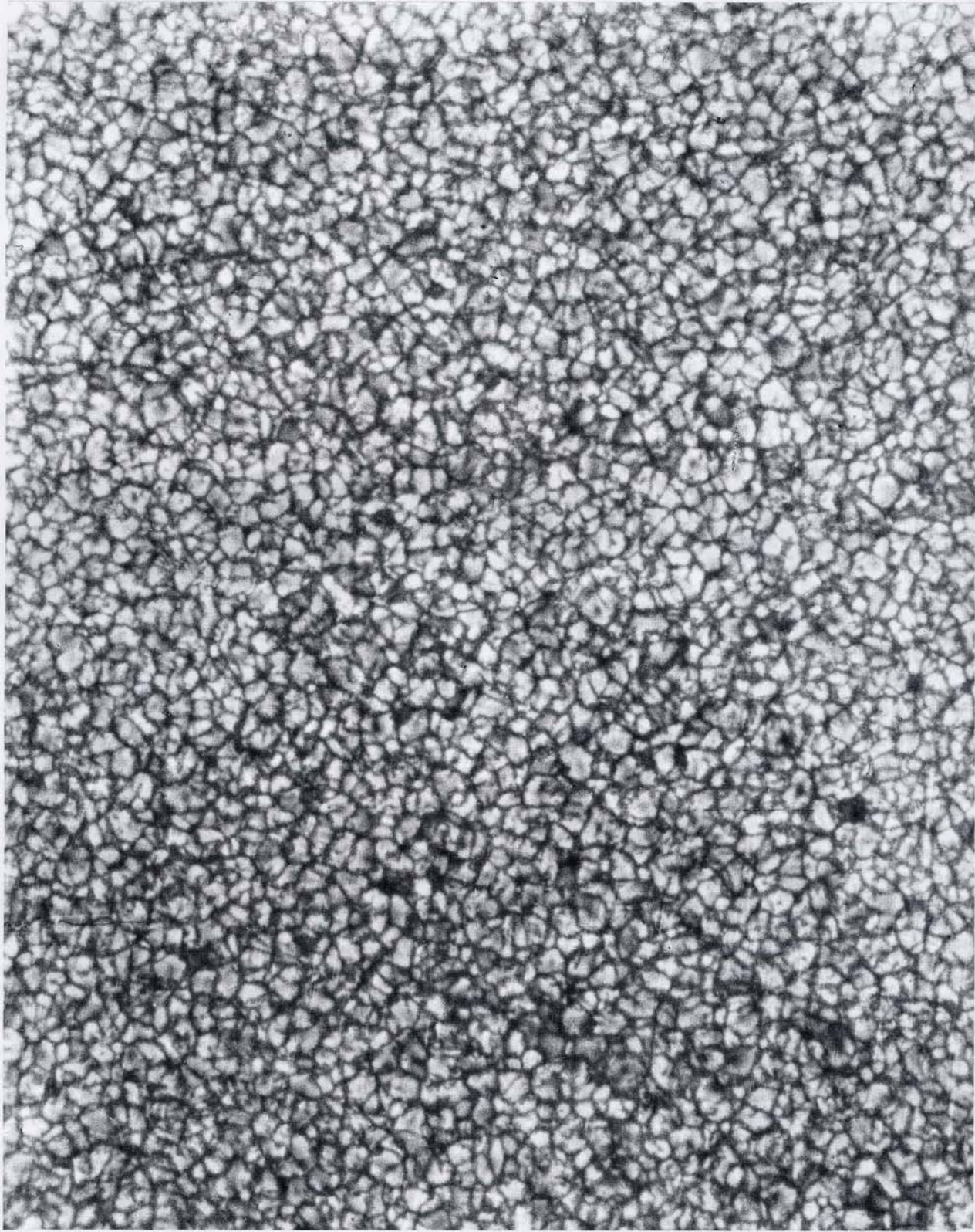
Турбулентная поверхность Солнца. Видна грануляция — чередование участков солнечной поверхности, где горячий газ поднимается или опускается. Каждая турбулентная ячейка имеет поперечник около 2000 км — примерно как расстояние от Парижа до Киева. Снимок в обычном желтом свете сделан в обсерватории Пик-дю-Миди, Франция.
