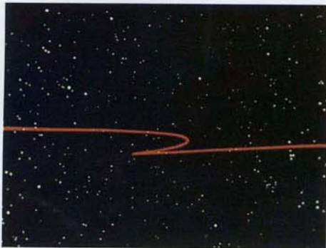
Попытное движение на многомесячном пути планеты Марс среди созвездий.
