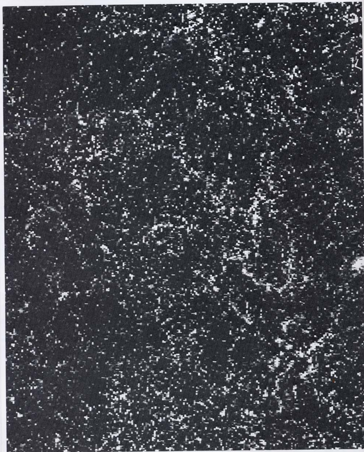
Крупномасштабная текстура Космоса: небольшой фрагмент карты, охватывающей миллионы ярчайших галактик на расстоянии до миллиарда световых лет от Земли. Каждый маленький квадратик — это галактика, содержащая миллиарды звезд. Карта построена по результатам телескопического обзора, который Доналд Шейн и Карл Виртанен из Ликской обсерватории Калифорнийского университета составляли 12 лет.
