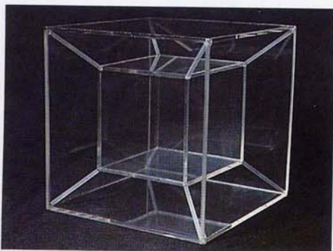
Обычное трехмерное изображение тессеракта или гиперкуба (эта трехмерная модель утратила одно из своих измерений при воспроизведении ее на странице книги).
