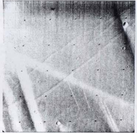
Необъясненные линейные структуры на Равнине Тарсис. Снимок «Маринера-9». С разрешения NASA
