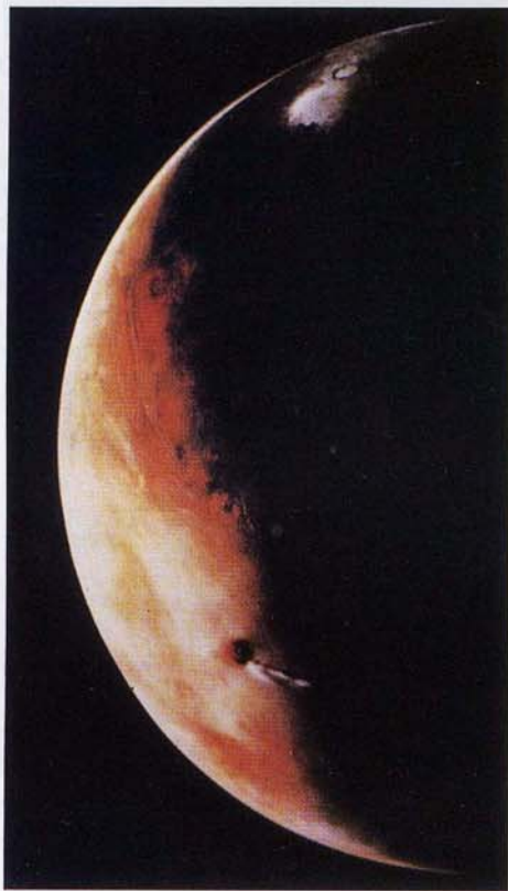
Далекая встреча: «Викинг» снимает марсианский серп. Видны кратер на Северной полярной шапке и высокогорные облака с подветренной стороны гигантского вулкана Олимп. С разрешения NASA
