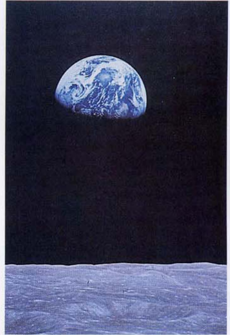
Земля над Луной: увидеть это мечтал Кеплер.
