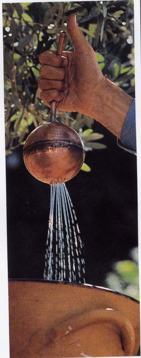
Современная реконструкция клеписидры, или «водяного вора», с помощью которой Эмпедокл обосновал, что воздух состоит из неисчислимых мельчайших частиц. Фото Б. Рэя
