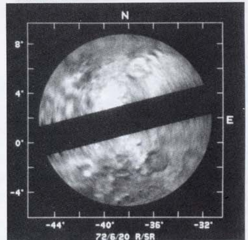
Детальное изображение области вблизи экватора Венеры, по данным радиолокации с Земли. Диагональная полоса — область, по которой не было получено данных. Видно несколько кратеров, крупнейший из них имеет в поперечнике почти 200 км. По сравнению со многими другими телами Солнечной системы кратеры на Венере очень мелкие, что указывает на работу механизмов эрозии. Станция слежения Голдстоун, Лаборатория реактивного движения, NASA
