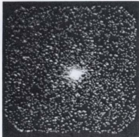
Рентгеновский снимок неба, на котором виден яркий источник, кандидат в черные дыры Лебедь X-1 (в центре). Снимок орбитальной обсерватории HEAO-2. С разрешения Р. Джаккони и NASA
