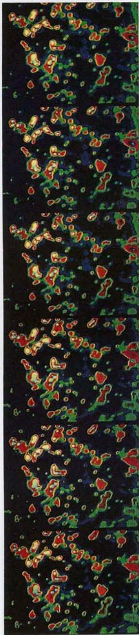
Атомы в движении: несколько последовательных кадров, запечатлевших возмущения углеродного фона (сине-черный) случайными движениями атомов урана (красные). Демокрит порадовался бы этому фильму. С разрешения А. Крюи, Чикагский университет
