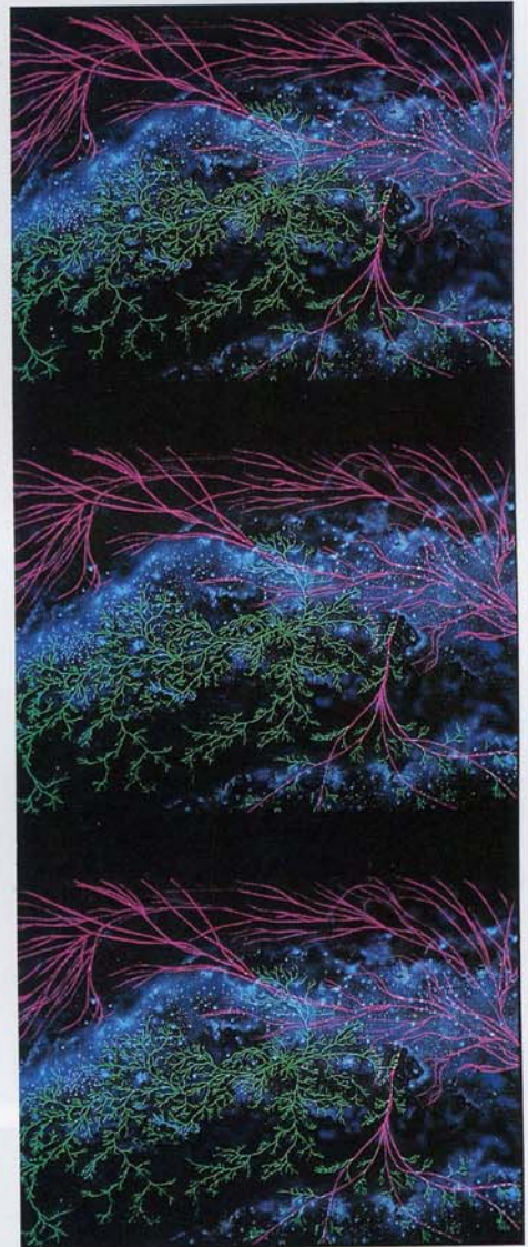
Межзвездная колониальная цивилизация, распространяющаяся от одной планетной системы к другой относительно короткими прыжками (зеленая), встречается с другой подобной цивилизацией (красная), но способной к более дальним путешествиям. Анимация Д. Якобсона
