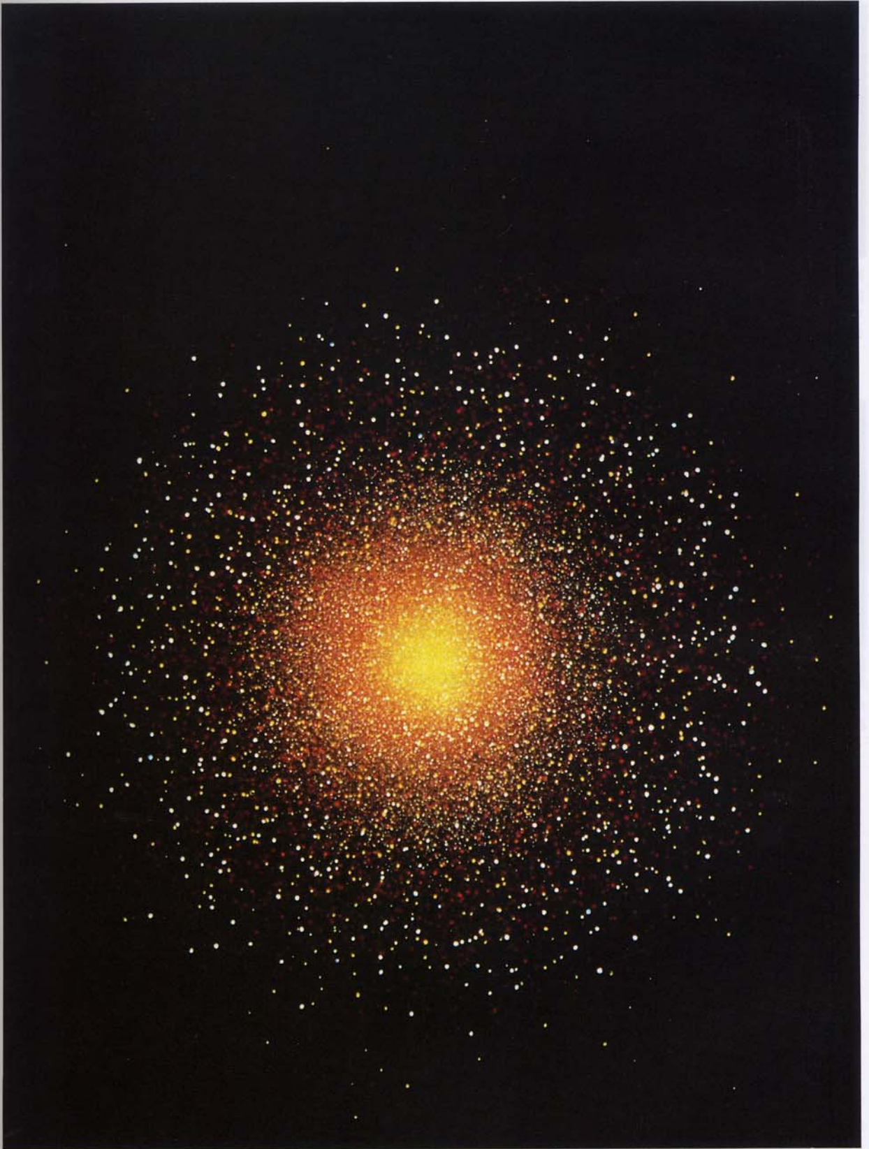
Шаровое звездное скопление, обращающееся вокруг ядра Галактики. Художник А. Норсиа
