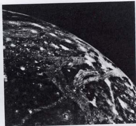
Ганимед — самый крупный из спутников Юпитера. Наименьшие различимые на этом снимке «Вояджера-1» детали имеют размер около трех километров. Видны многочисленные ударные кратеры с яркими лучами. Происхождение слегка изогнутых пересекающихся полос, состоящих из параллельных борозд, не выяснено. С разрешения NASA
