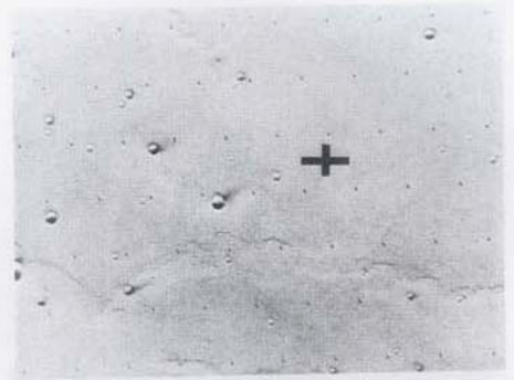
Спокойный рельеф Равнины Хриза в районе посадки «Викинга-1». После перелета длиной в сотни миллионов километров касание поверхности произошло в нескольких километрах от намеченной точки, обозначенной крестом. С разрешения NASA
