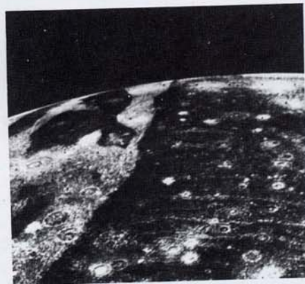
Снимок Ганимеда, сделанный 8 июля 1979 г. «Вояджером-2». Светлые параллельные полосы, протянувшиеся поперек темной равнины (справа), могли появиться на ледяной поверхности, подобно ряби на воде, в момент давнего ударного события. Однако в предполагаемом месте столкновения нет кратера, возможно из-за медленных вязких деформаций на протяжении огромного времени. С разрешения NASA
