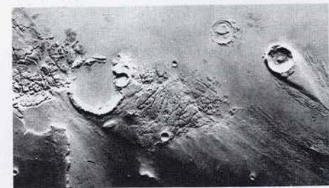
Покрытая кратерами местность вблизи Бассейна Хриза в давние времена была залита потоками воды. Это одна из причин, по которой Хризу выбрали для посадки «Викинга-1», однако по соображениям безопасности точное место посадки оказалось немного в стороне от самого Бассейна. С разрешения NASA
