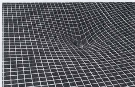
Схематическое изображение искривления плоского пространства массивным объектом, полезное для понимания гравитации и черных дыр.
