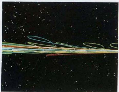
Видимое движение нескольких планет на одном участке неба на протяжении месяцев.
