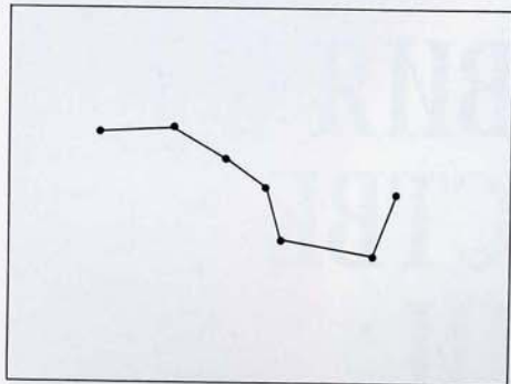
Большая Медведица, видимая с Земли
