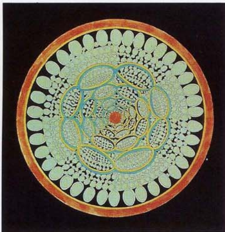
Условное изображение высокоразвитой технической цивилизации, которая перестроила свою планетную систему в сферическую оболочку, окружающую центральную звезду, так что большая часть ее ценного излучения не теряется в космосе. Художник Дж. Ломберг
