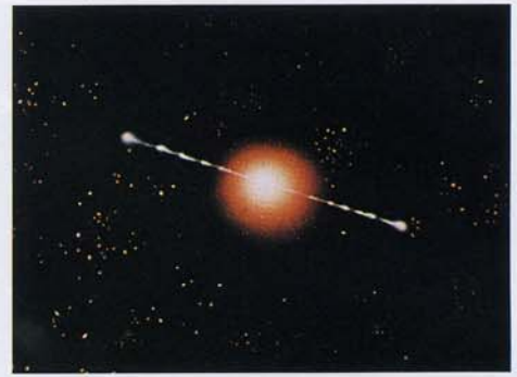
Взрывающаяся радиогалактика с двумя симметричными выбросами — джетами. Художник А. Шеллер
