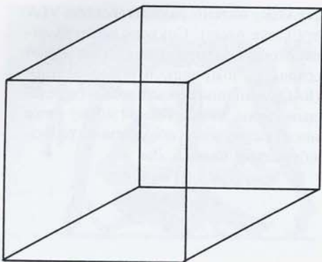
Обычное двумерное изображение куба.
