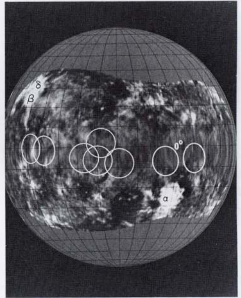
Радарная карта экваториального пояса Венеры. Светлые области эффективно отражают радиоволны обратно в космос. Окружностями отмечены области, исследованные более подробно, одна из них показана на следующем рисунке. Подробная карта Венеры представлена на с. 358. Станция слежения Голдстоун, Лаборатория реактивного движения, NASA
