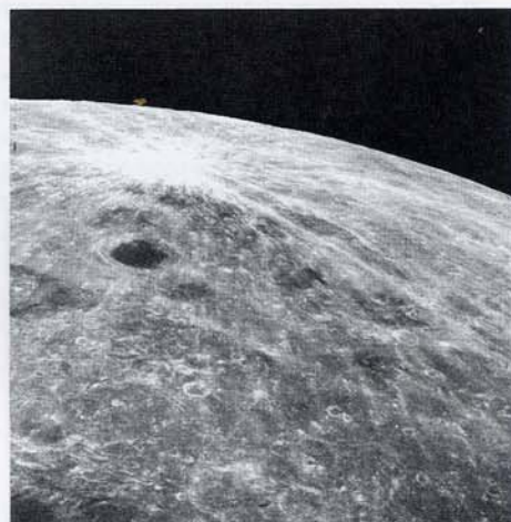
Лучистый кратер Бруно (вверху) на поверхности Луны. Снимок с орбитального модуля «Аполлона». С разрешения NASA
