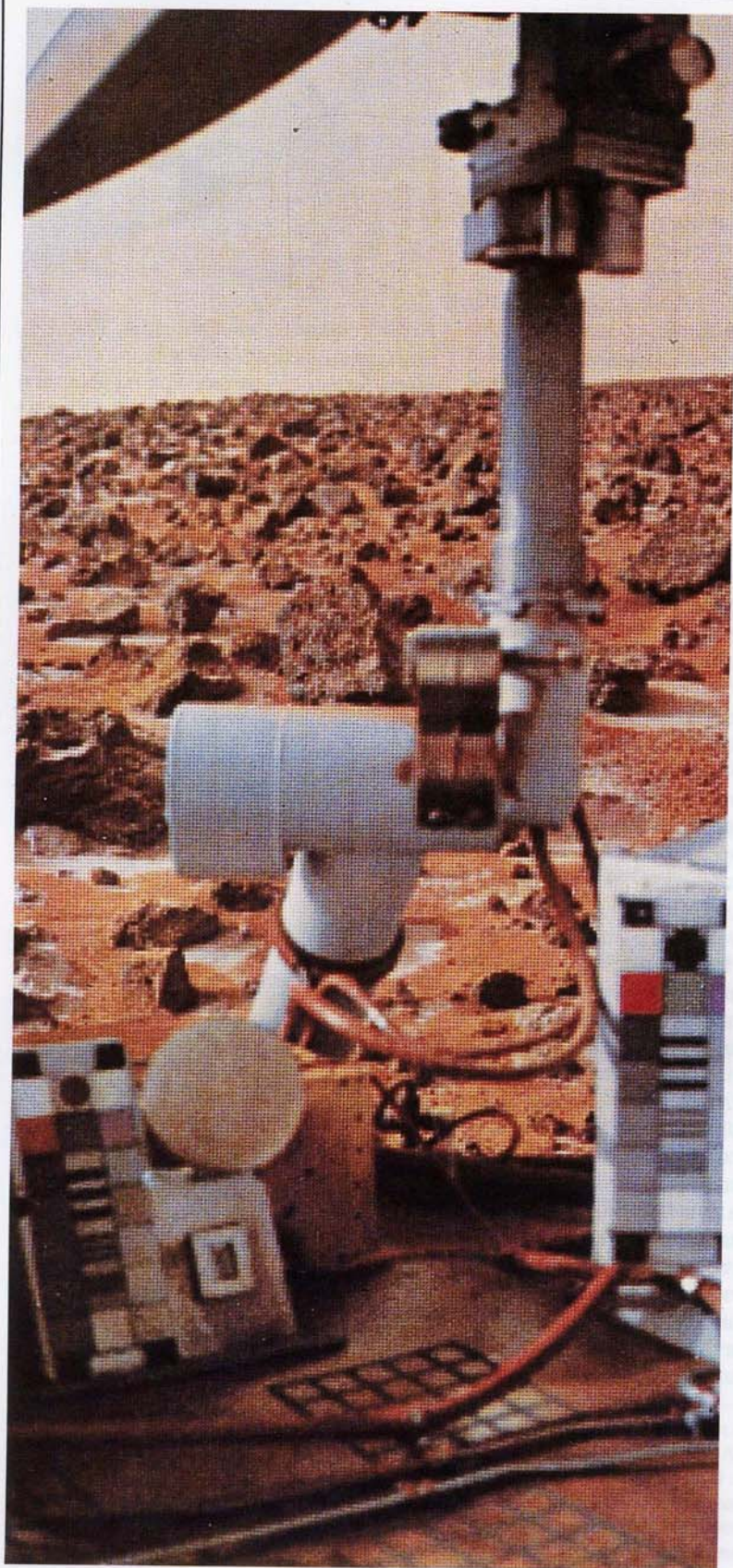
Иней в Утопии. На 44^{\circ} с. ш. Марса в октябре 1977 г.: тонкий слой водяного инея покрывает грунт в начале северной зимы. Вертикальная конструкция поддерживает остронаправленную антенну «Викинга-2» для прямой связи с Землей. Цветные квадраты и черные полосы — это калибровочные мишени для камеры. Черный квадрат с белым контуром внизу слева — микрофиса, на которой изображены (очень мелко) подписи десяти тысяч человек, участвовавших в конструировании, изготовлении, тестировании и запуске космического аппарата «Викинг». Люди, почти не замечая того, становятся мультипланетным видом. С разрешения NASA
