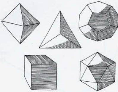
Пять правильных пифагоровых (или платоновых) тел (см. Приложение 2)
