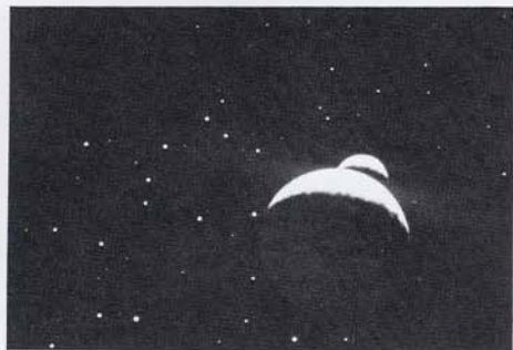
Плутон, покрытый метановой корой, и его спутник Харон. Художник Дж. Оллисон
