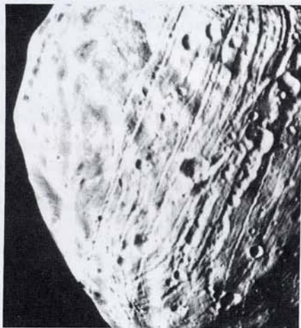
Детальный снимок системы борозд на Фобосе, порожденных, возможно, приливным воздействием со стороны Марса. На поверхности Фобоса и его брата Деймоса, по видимому, имеется значительное количество органического вещества, которое придает им темный цвет. Оба они могут быть захваченными астероидами. Размеры этого крошечного спутника составляют 27 \times 21 \times 19 км, причем длинная ось направлена в сторону Марса. Снимок с орбитального аппарата «Викинг-1». С разрешения NASA
