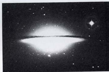
Галактика Сомбреро, М104 (также обозначаемая NGC 4594). Спиральные рукава, прослеживаемые по полосе пыли, плотно охватывают ядро из звезд. Галактика расположена примерно в 40 млн. световых лет от нас, гораздо дальше, чем окружающие звезды созвездия Девы, и может содержать около триллиона звезд. Наша галактика Млечный Путь будет выглядеть похоже, если наблюдать ее с ребра и примерно с такого же расстояния. С разрешения Обсерватории Хейла
