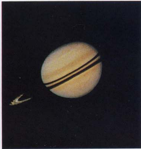
Снимок Сатурна и его колец, сделанный «Пионером-11» с расстояния 2,5 млн. км 29 августа 1979 г., после более чем пятилетнего полета. С разрешения NASA
