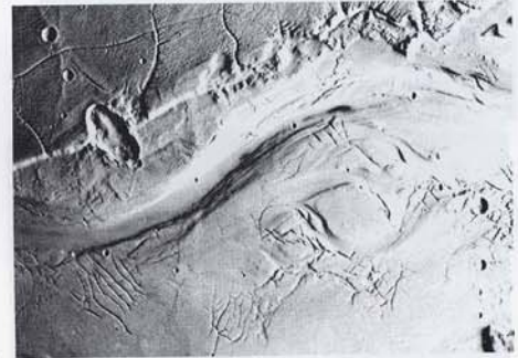
Участок Долины Касэй, древней речной долины на Марсе. «Касэй» — так по-японски называется Марс. Ударные кратеры на дне русла свидетельствуют о его солидном возрасте. Значительное количество воды на поверхности Марса в далеком прошлом говорит о том, что когда-то условия здесь подходили для жизни гораздо больше. Снимок с орбитального модуля «Викинга». С разрешения NASA
