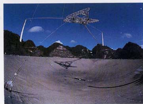
Радарная радиообсерватория Аресибо в Пуэрто-Рико. Над полусферической отражающей тарелкой нависает рупор, поддерживаемый тремя мачтами, две из которых на нижнем снимке выглядят изогнутыми из-за использования камеры с объективом «рыбий глаз», установленной на поверхности тарелки. Фото Б. Рэя. С разрешения Национального астрономического и ионосферного центра, Корнеллский университет
