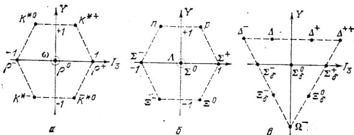
Рис. 20. Октект векторных мезонов с единичным спином (а), октект барионов со спином 1/2 и положительной пространственной четностью (б); декуплет барионов со спином 3/2 и положительной пространственной четностью (в)
