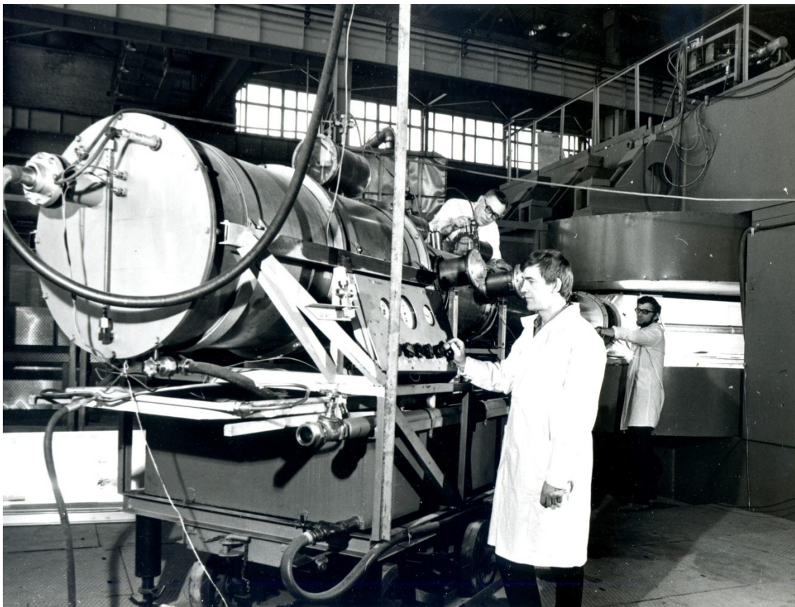
Монтаж генератора на 500 кV в измерительном павильоне СФ
