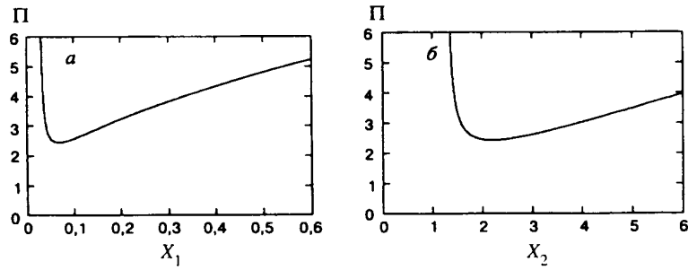
Рис.14. Зависимость параметра подобия Π от X_1 (a) и X_2 (б) в случае кумулятивной кинематики
