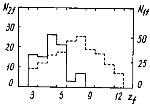
Рис.2. Распределение по заряду f_2 -фрагментов в 2f -событиях с Z_{f1}=3 — сплошная гистограмма (а); фрагментов с Z \geq 3 в 1f -событиях — штриховая гистограмма (б).
