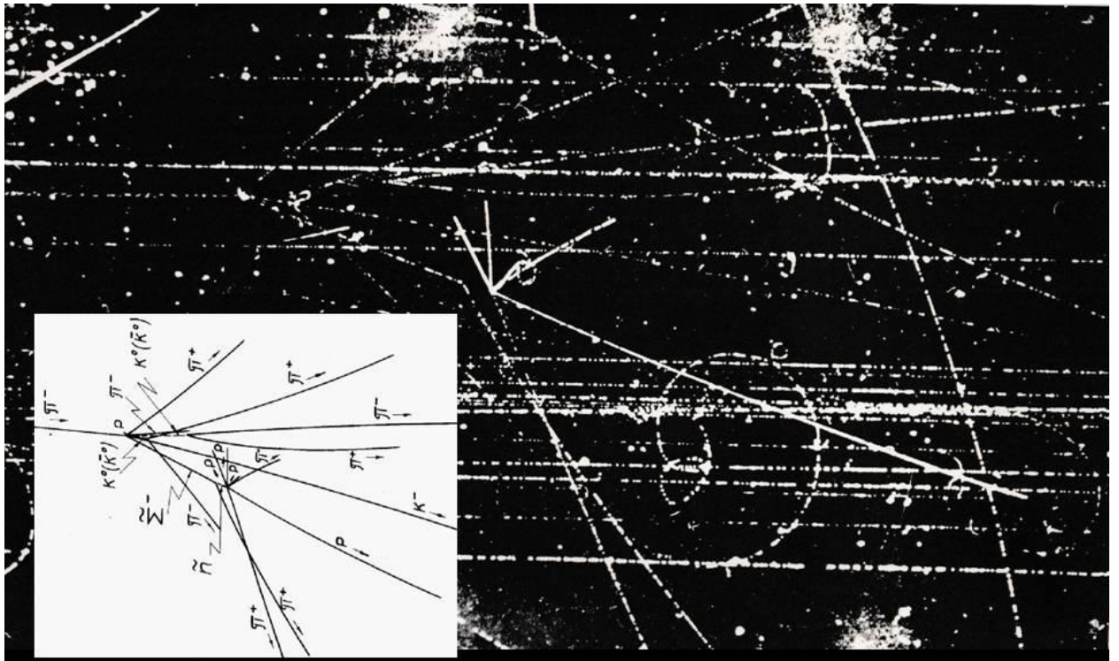
Рис. 9. Фотография в пузырьковой камере образования и распада анти- \Sigma^- -гиперона на антинейтрон, проявившийся в звезде аннигиляции и \pi^+ -мезон (предоставлено А.А. Кузнецовым).
