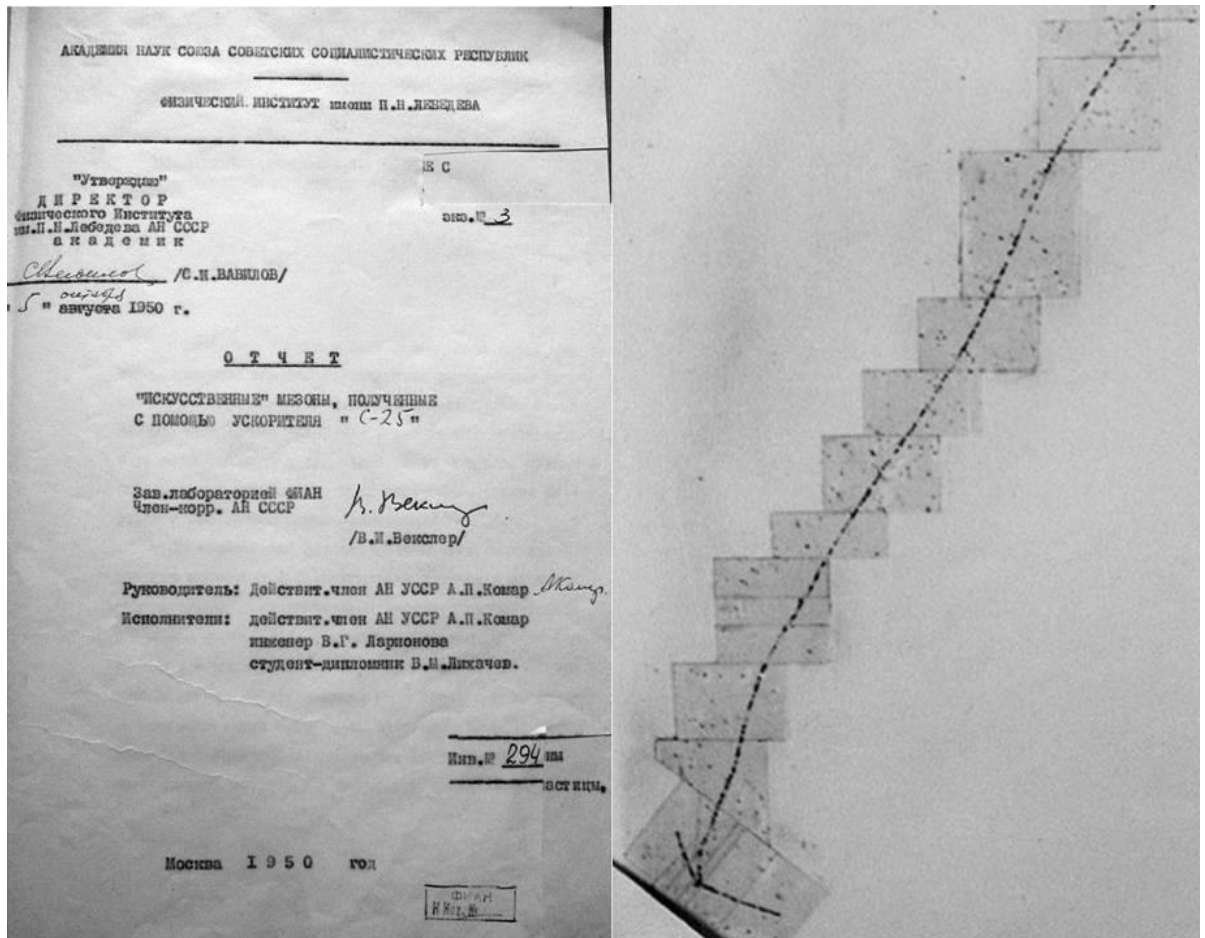
Рис. 1. Титульная страница отчета ФИАИ и фотография извилистого следа \pi^- -мезона, захваченного ядром эмульсии с образованием двух фрагментов (предоставлено С.П. Харламовым).
