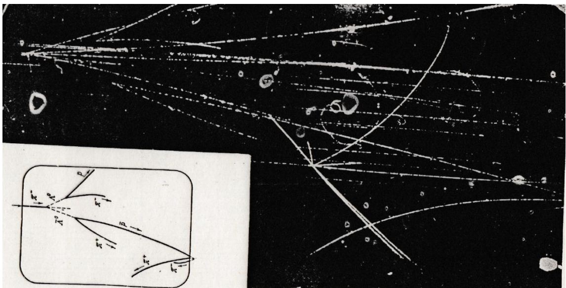
Рис. 8. Фотография в пузырьковой камере редкого события - образования и распадов пары \Lambda и анти- \Lambda -гиперонов (предоставлено А.А. Кузнецовым).
