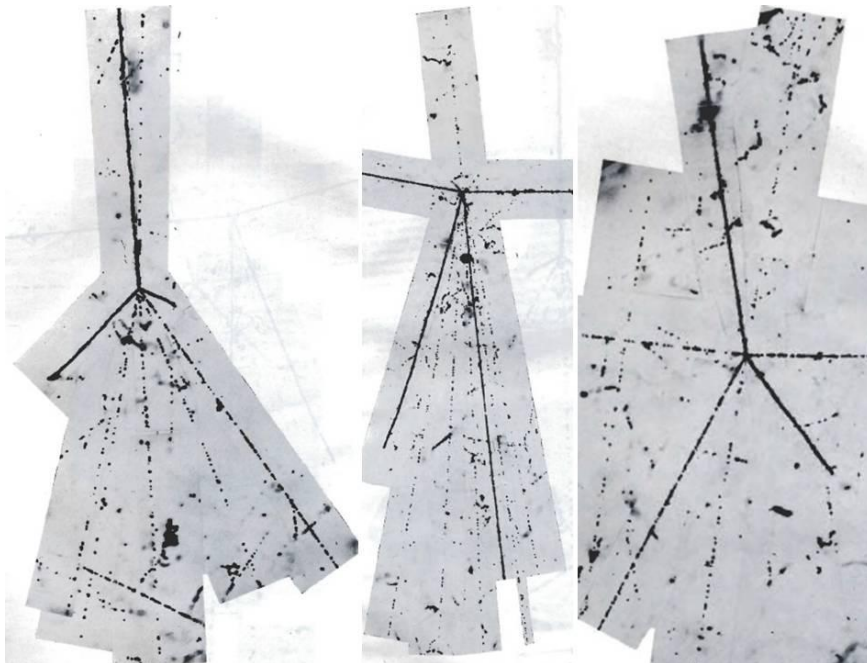
Рис. 5. Макрофотография взаимодействия ядра космического происхождения в ядерной эмульсии (ФИАН, начало 50-х гг, предоставлено Г.И. Орловой).
