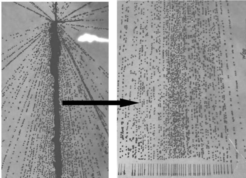
Рис. 5. Макрофотография взаимодействия ядра космического происхождения в ядерной эмульсии (ФИАН, начало 50-х гг, предоставлено Г.И. Орловой).
