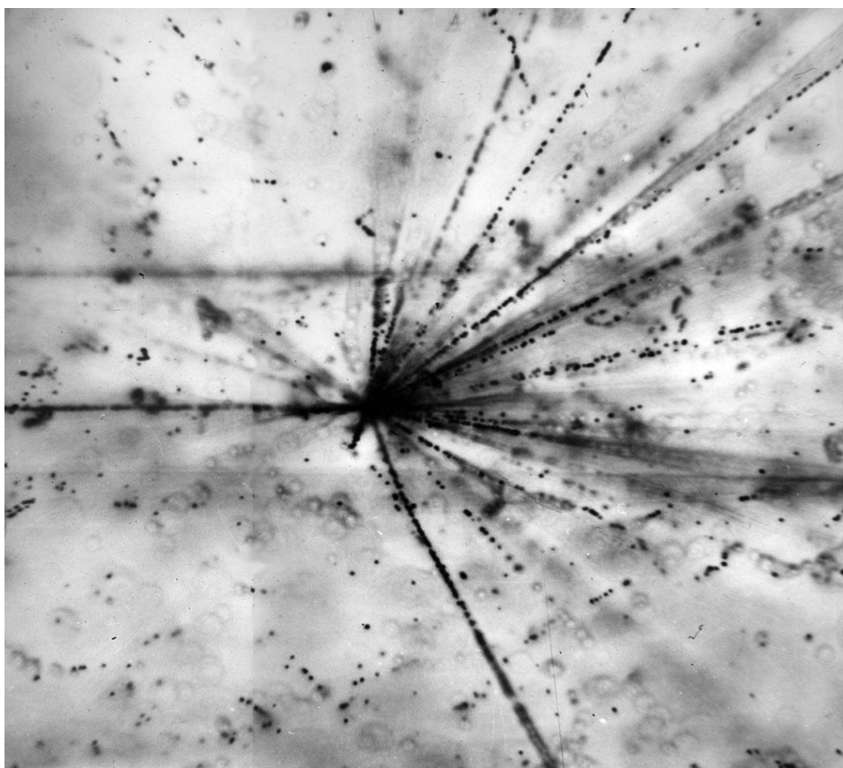
Рис. 12. Фотография центрального соударения ядра ^{12}\text{C} с энергией 3.65 ГэВ на нуклон в ядерной эмульсии (предоставлена К. Д. Толстовым).
