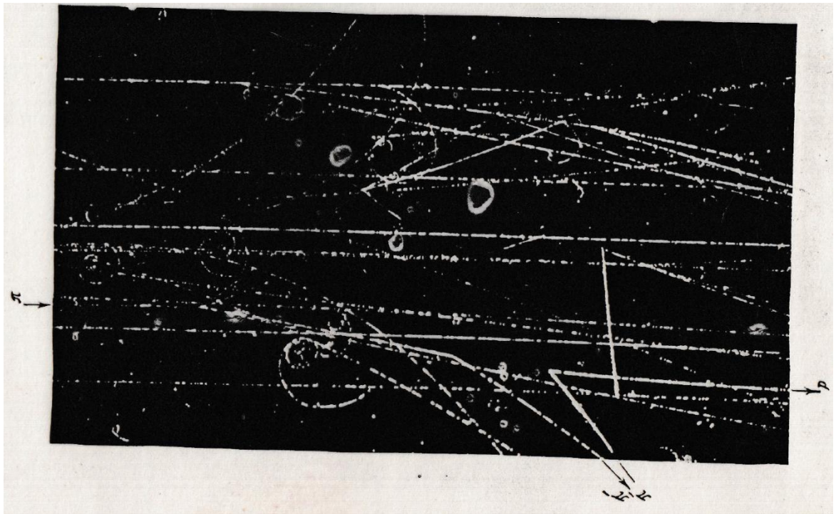
Рис. 7. Фотография в пузырьковой камере образования \Xi^- -гиперона распадающегося на пару \Lambda\pi^- (предоставлено А.А. Кузнецовым).
