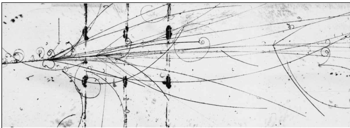
Рис. 13. Фотография центрального соударения ядра ^{12}\text{C} с энергией 3.65 ГэВ на нуклон в пропановой пузырьковой камере (предоставлена М. И. Соловьевым).
