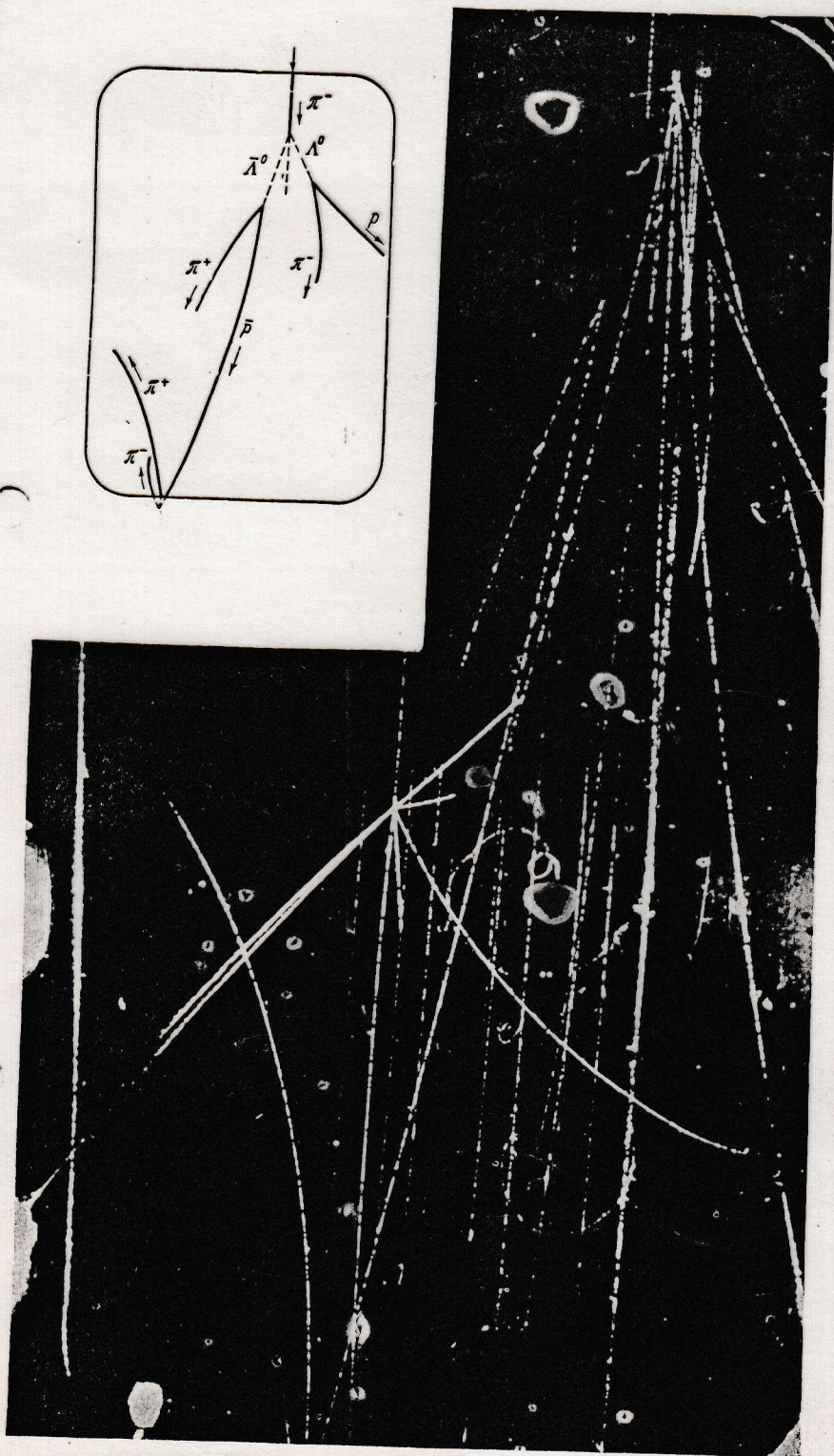
Фотография события, на которой виден случай рождения и распада \bar{\Lambda} + \Lambda -гиперонов и схема события
